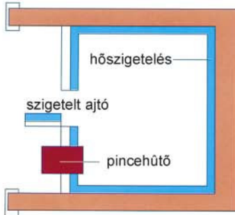
Beépítési példa a Wine C típusra
