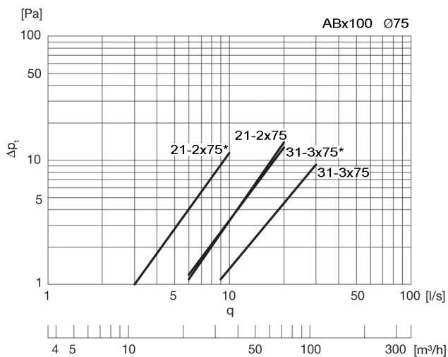
Befúvás / elszívás (a nyomásesés görbék SZR szellőzőráccsal együtt értendőek)
